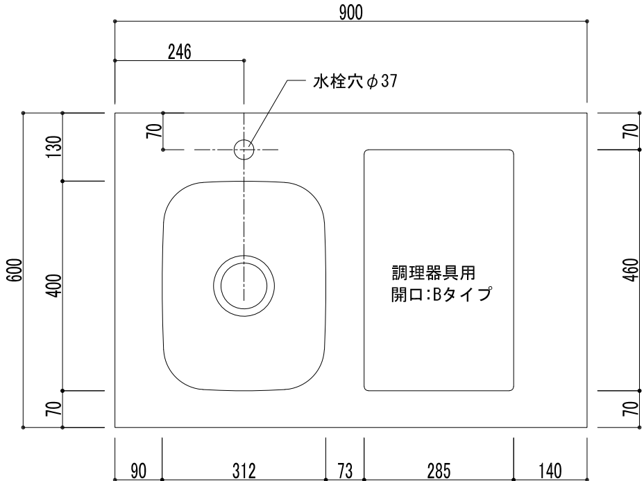
平面図
